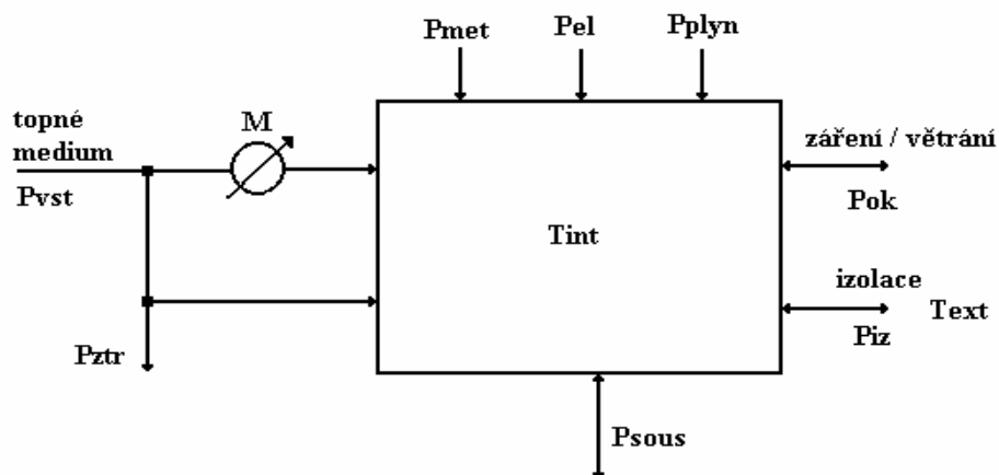
Obr.1. Schéma tepelných toků jednoho bytu.
