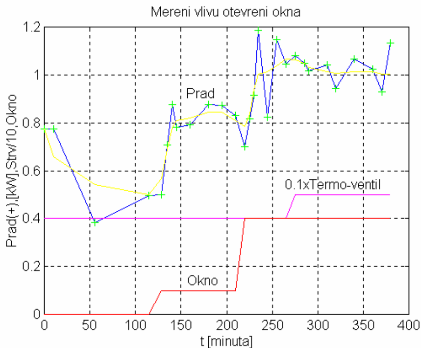
Obr.4. Záznam měření vlivu otevření větráčky nad radiátorem.
