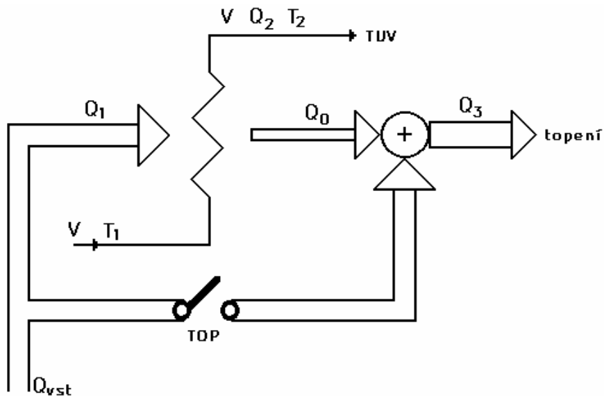
Obr.3. K výpočtu ceny TUV.
