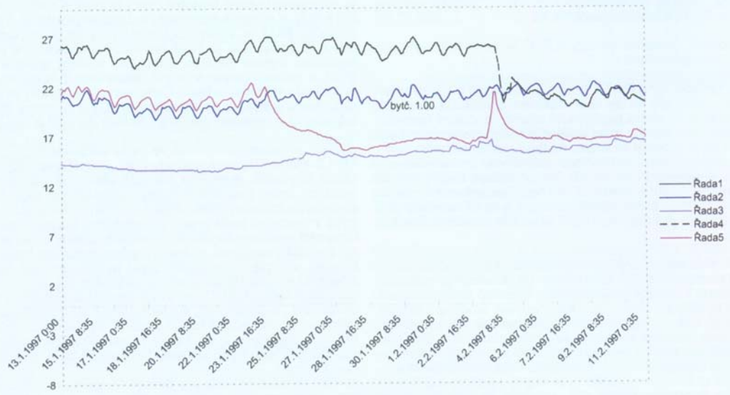
Průběh teplot v bytech č.1.00, č.1.01, č.1.14, č.1.20 - Brno, Bulharská ul.
